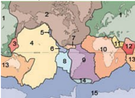
Tektonische Platten: 1 Eurasische, 2 Nordamerikanische, 3
